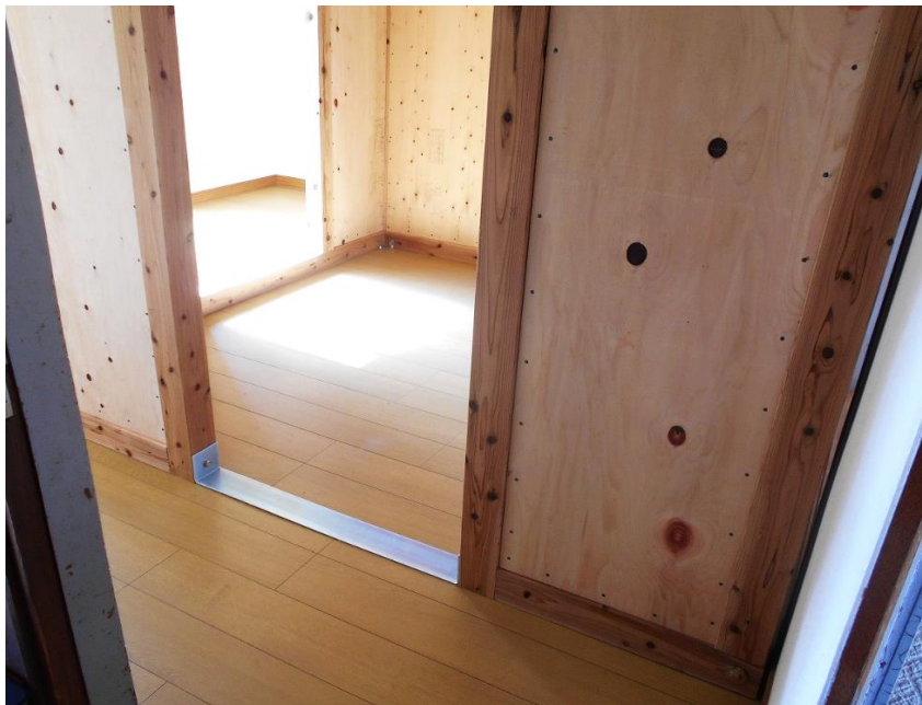
耐震シエルター組立
